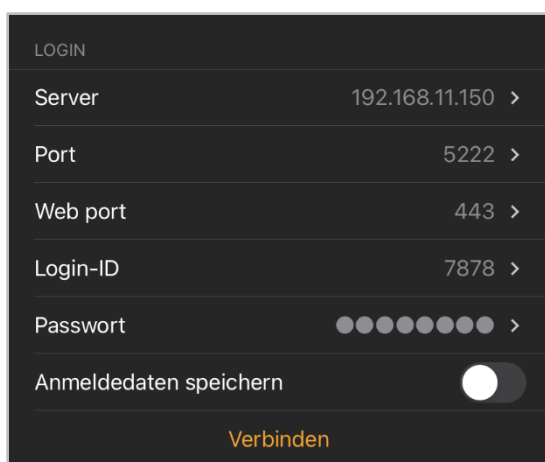
Abbildung 16 – Login-Einstellungen
